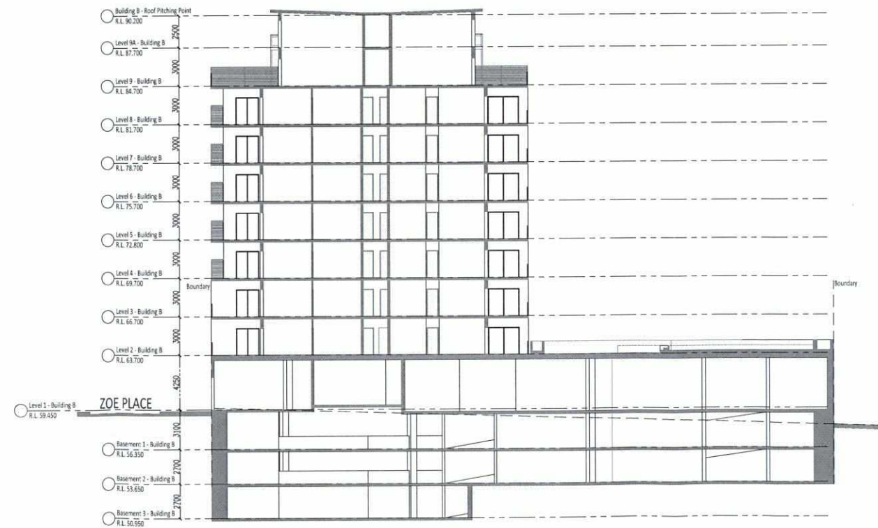
SECTION D-D
